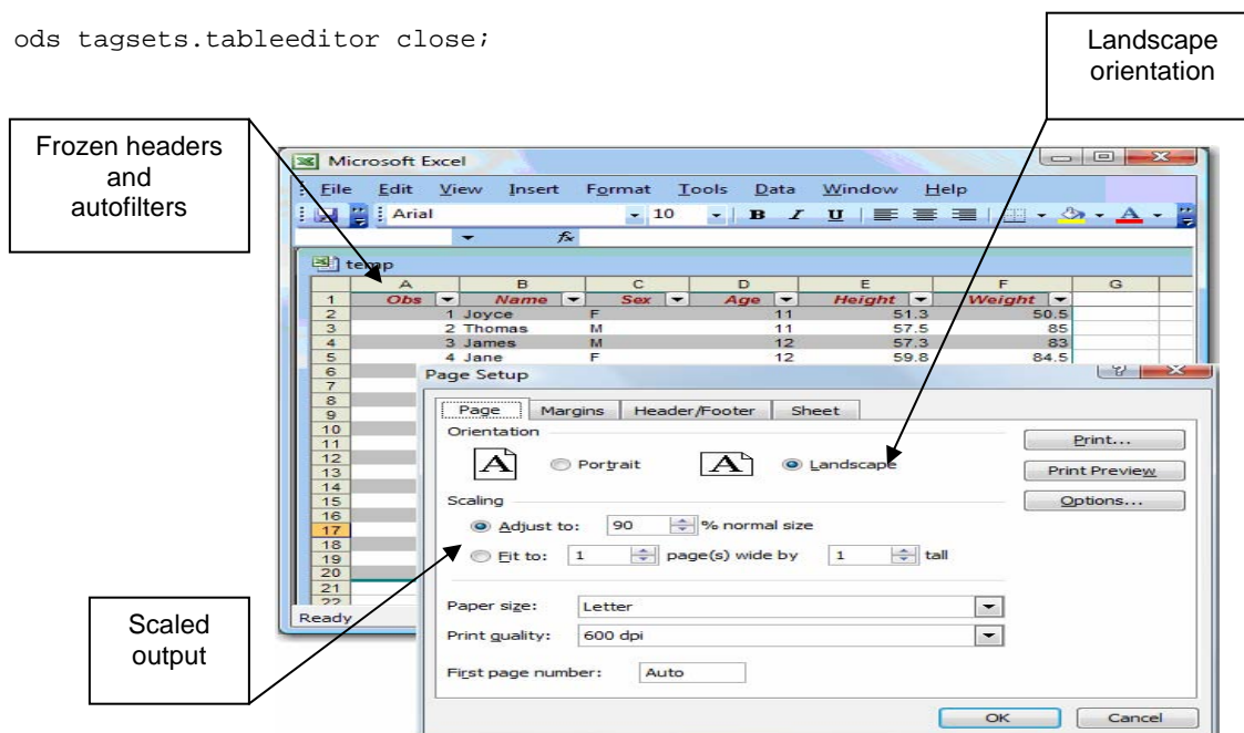
Display 30. Enhanced Output
