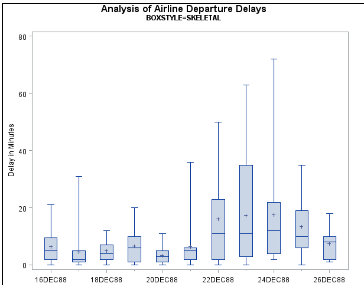
Output 24.3.1 BOXSTYLE=SKELETAL
