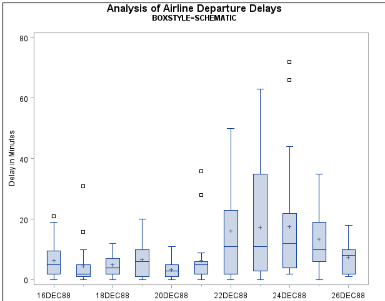
Output 24.3.2 BOXSTYLE=SCHEMATIC
