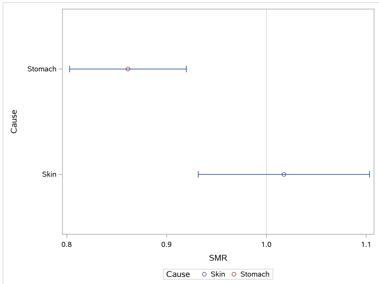
Output 113.4.10 SMR Results
