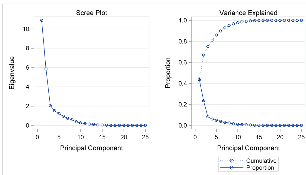
Output 94.1.1 Eigenvalue Plot
