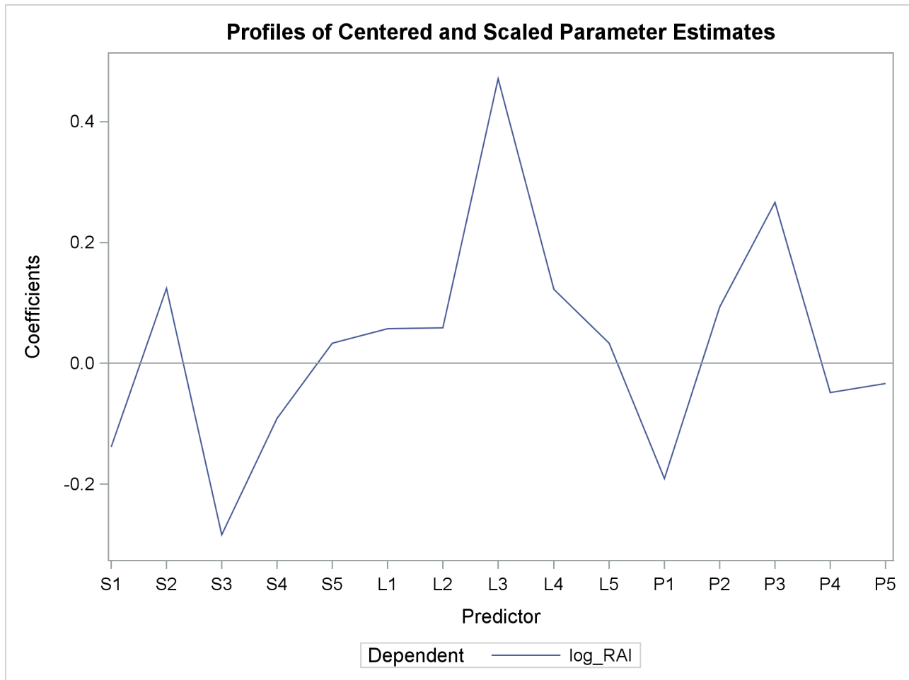
Output 74.1.6 Regression Parameter Profile
