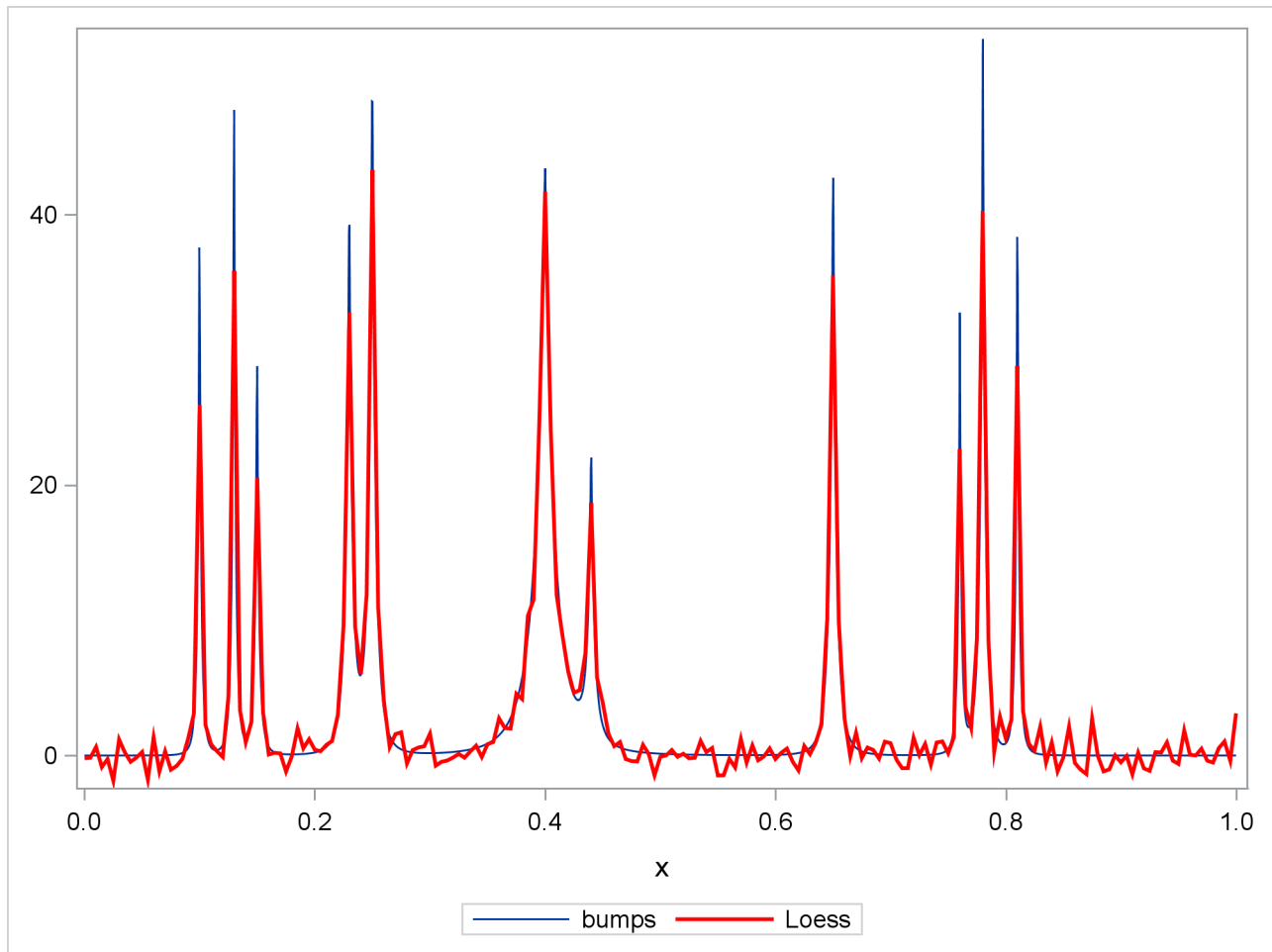
Output 47.3.2 Loess Fit
