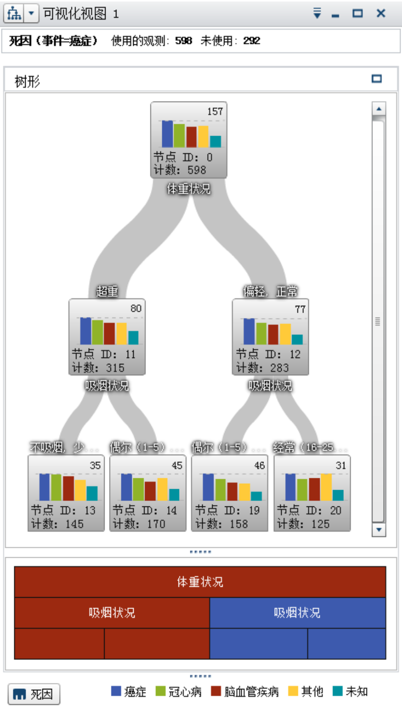
图 25.6 决策树示例
