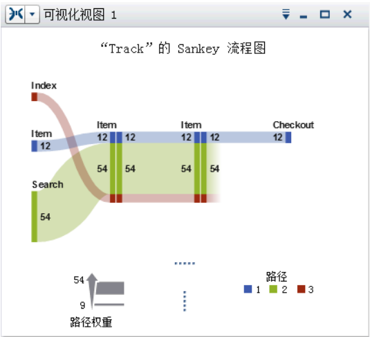
Sankey 流程图
