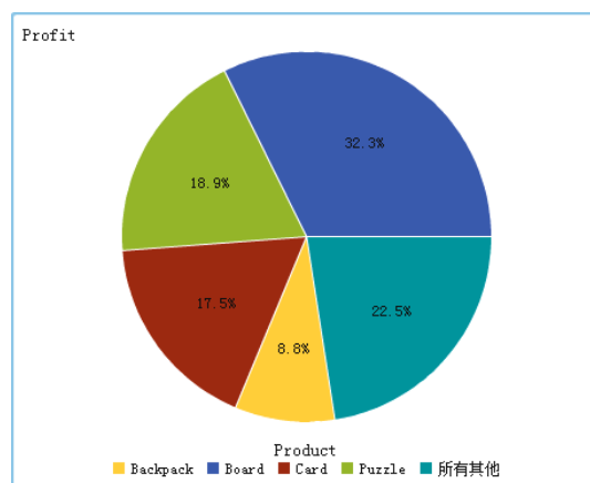
图 A2.7 饼图
