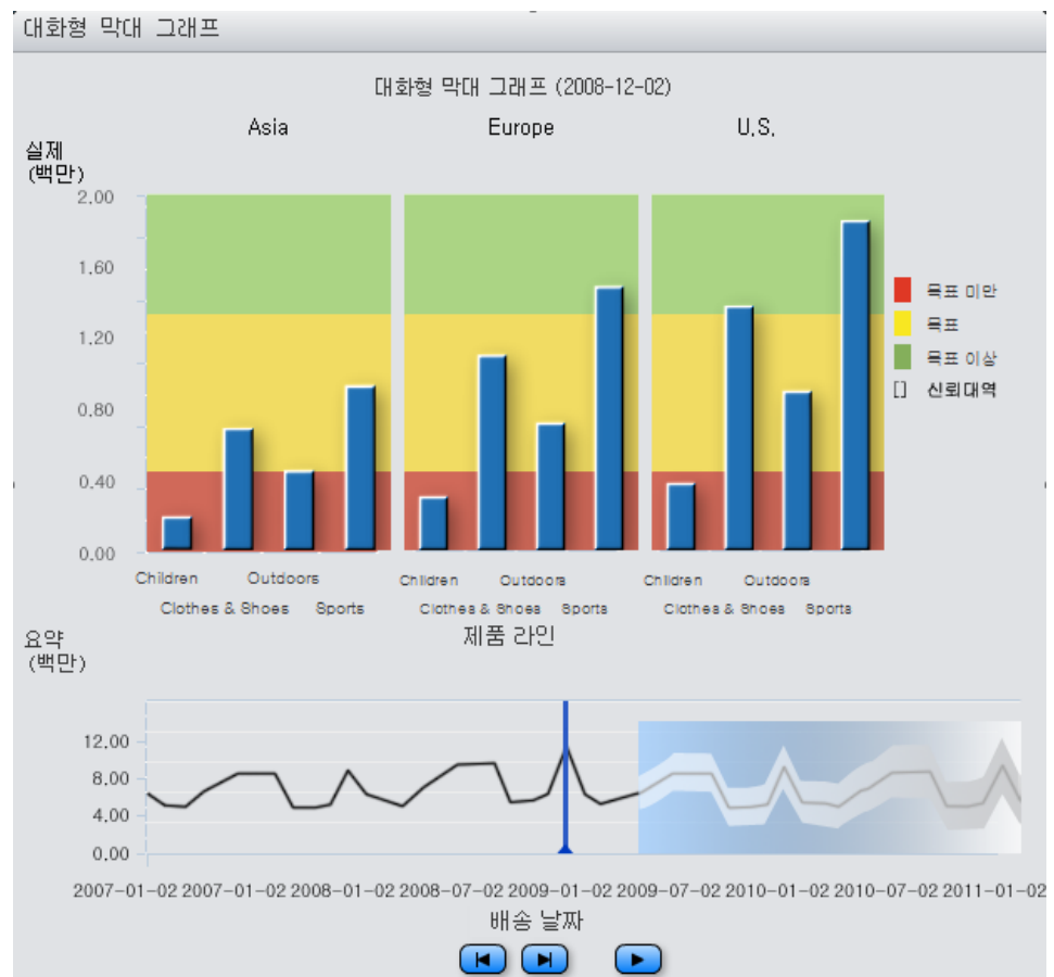
그림 A1.11 대화형 요약 및 막대 그래프 지표 예
