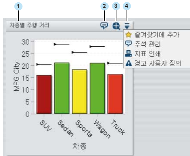
그림 4.3 지표 인터페이스
