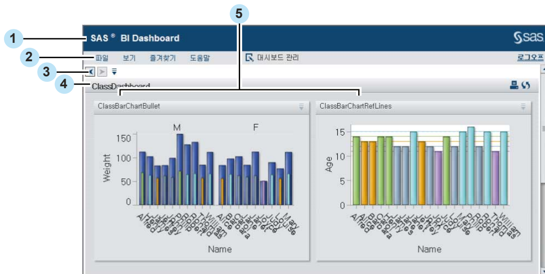
그림 4.2 대시보드가 표시된 SAS BI Dashboard 뷰어 인터페이스
