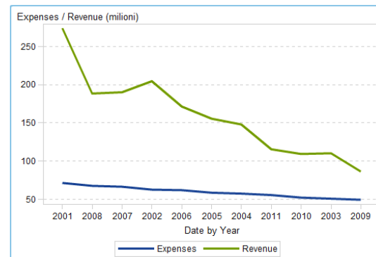
Figura A2.6 Grafico a linee
