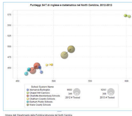
Figura A2.14 Diagramma di variazione a bolle
