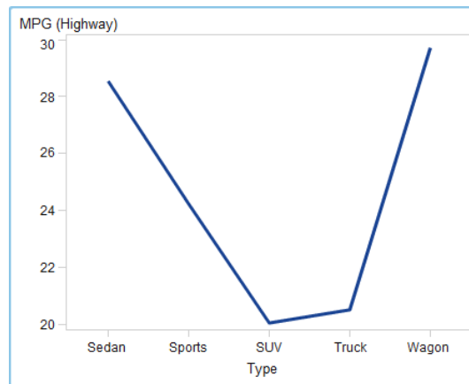
Figura A2.11 Diagramma della serie
