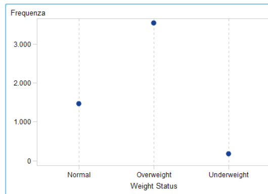
Figura A2.25 Diagramma a punti
