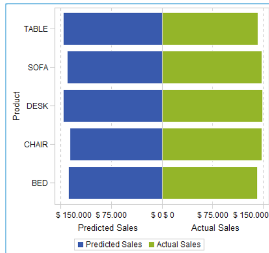
Figura A2.26 Grafico a farfalla
