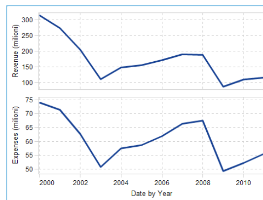
Figura A2.10 Grafico comparativo delle serie storiche
