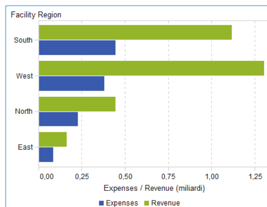
Figura A2.3 Grafico a barre
