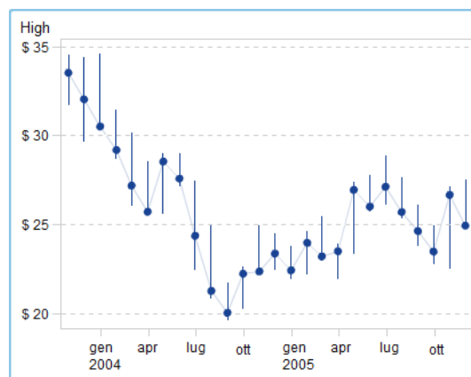
Figura A2.27 Diagramma max-min titoli
