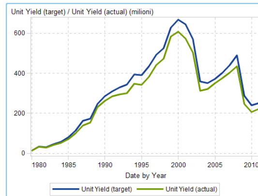
Figura A2.9 Grafico delle serie storiche
