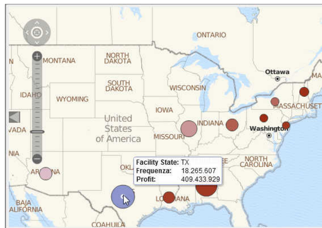
Figura A2.34 Mappa geo a bolle
