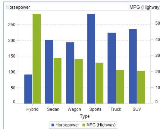
Figura A2.16 Grafico a barre con due assi
