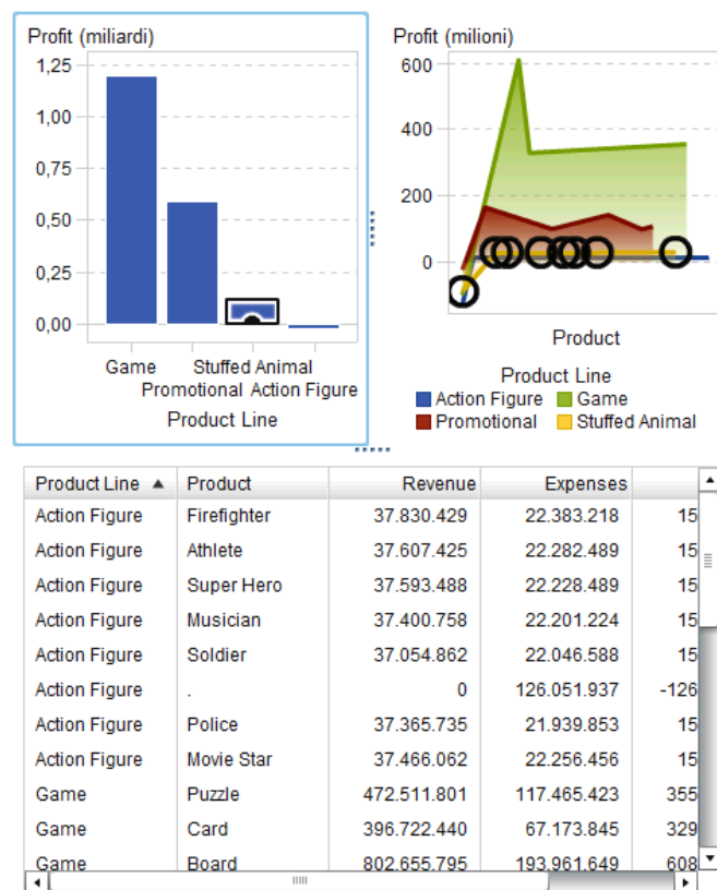
Figura 46.2 Esempio di evidenziazione interattiva dei dati con un grafico a barre, un grafico a linee e una tabella a elenco
