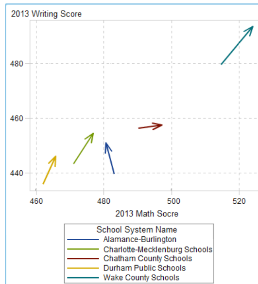
Figura A2.24 Diagramma vettoriale
