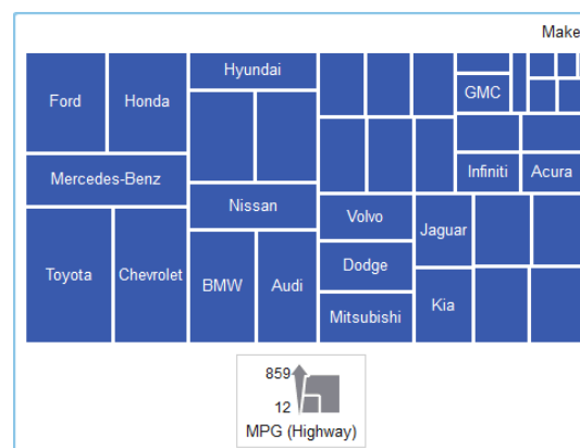
Figura A2.15 Grafico a mosaico
