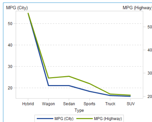
Figura A2.17 Grafico a linee con due assi
