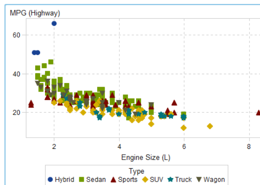
Figura A2.8 Grafico a dispersione
