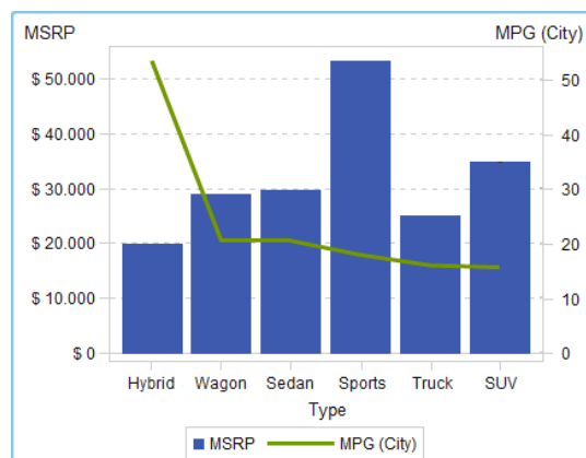
Figura A2.18 Grafico a barre e linee con due assi
