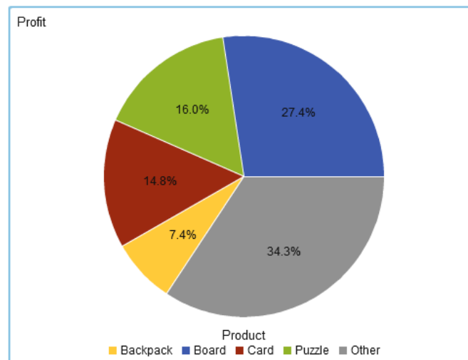
Figura 48.1 Grafico a torta con profitti per ogni linea di prodotti visualizzata
