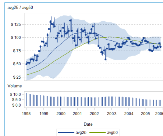
Figura A2.28 Diagramma di volatilità e volume titoli
