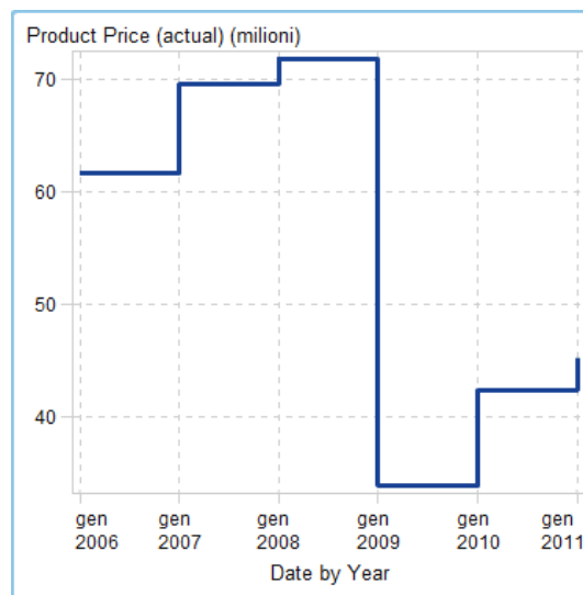
Figura A2.22 Grafico a gradino
