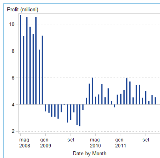
Figura A2.21 Diagramma ad aghi
