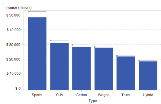
Figura A2.4 Grafico a barre con target
