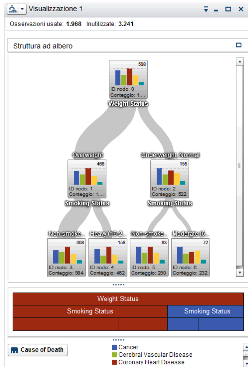
Figura 25.6 Albero decisionale di esempio
