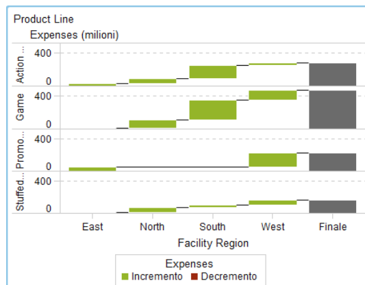
Figura A2.5 Grafico a cascata
