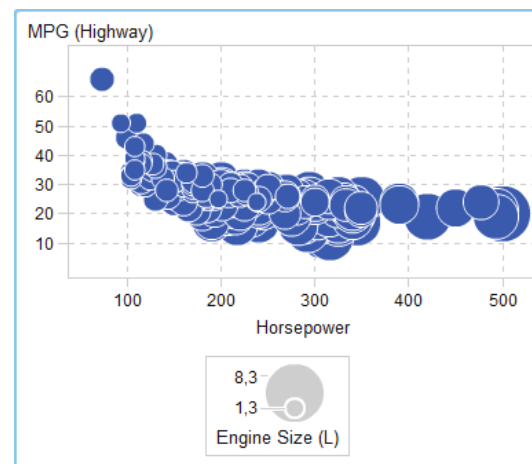
Figura A2.13 Grafico a bolle
