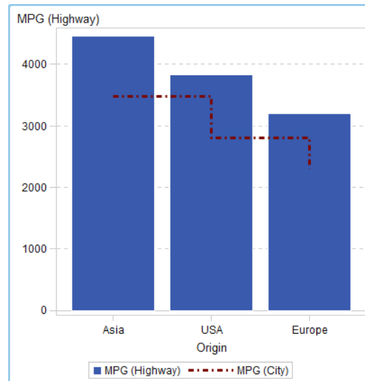
Figura 52.1 Grafico a gradino sovrapposto a un grafico a barre
