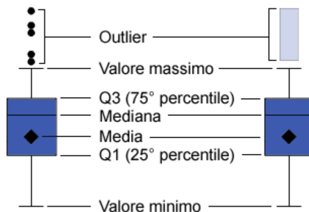
Figura 25.5 Parti di un box plot
