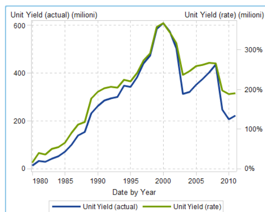
Figura A2.19 Grafico delle serie storiche con due assi
