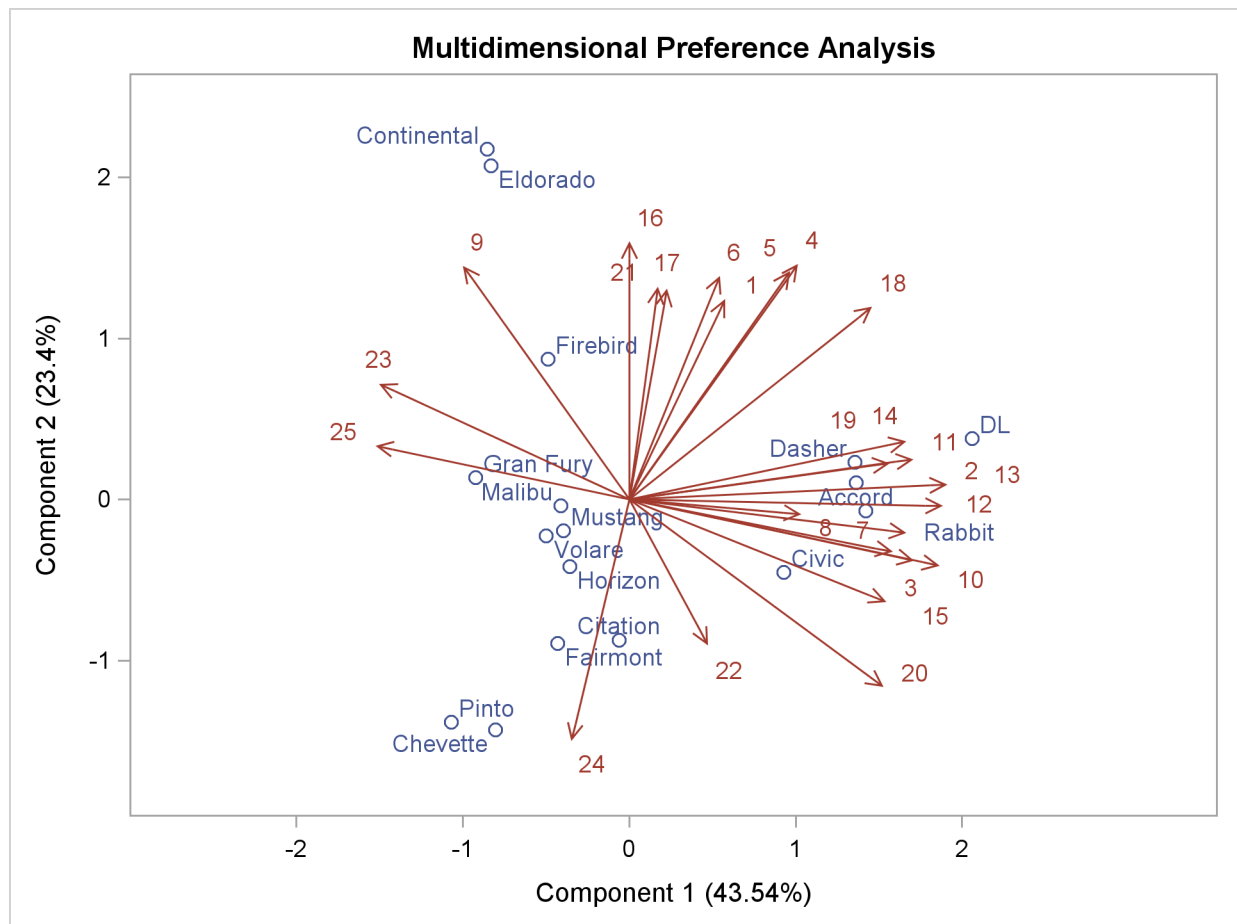
Output 90.6.2 MDPREF Plot
