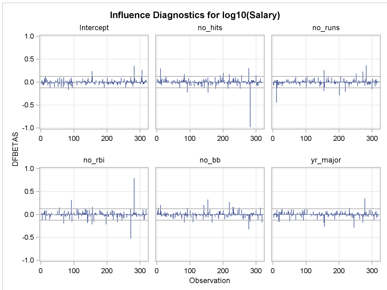
Output 73.1.15 DFBETAS
