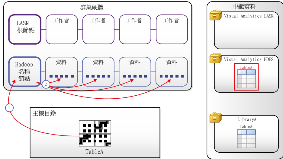
圖表 5.6 從共用的 HDFS 載入
