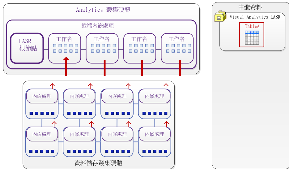
圖表 5.4 遠端平行載入
