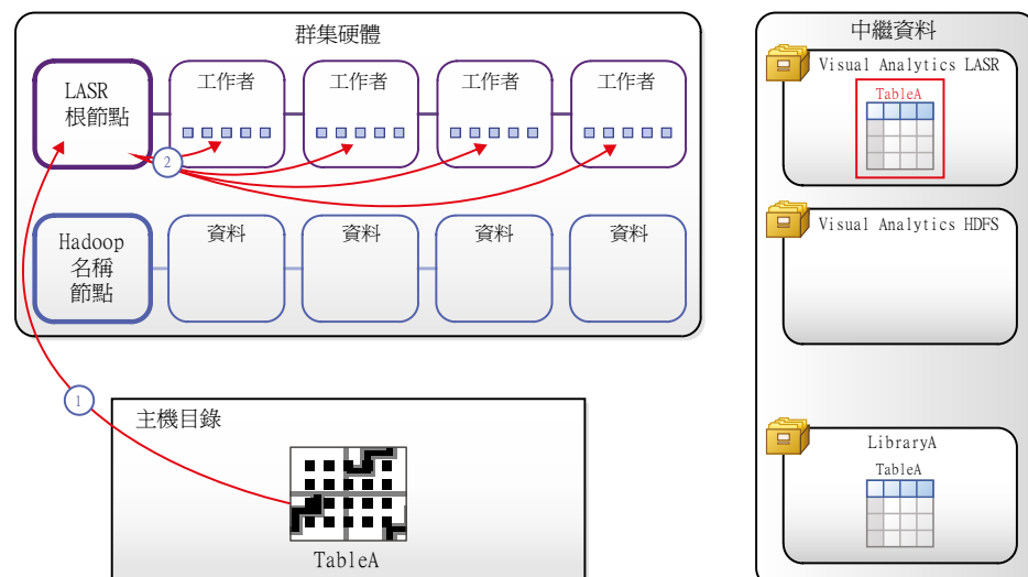
圖表 5.3 序列載入到分散式伺服器
