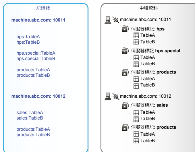
圖表 5.2 唯一性需求
