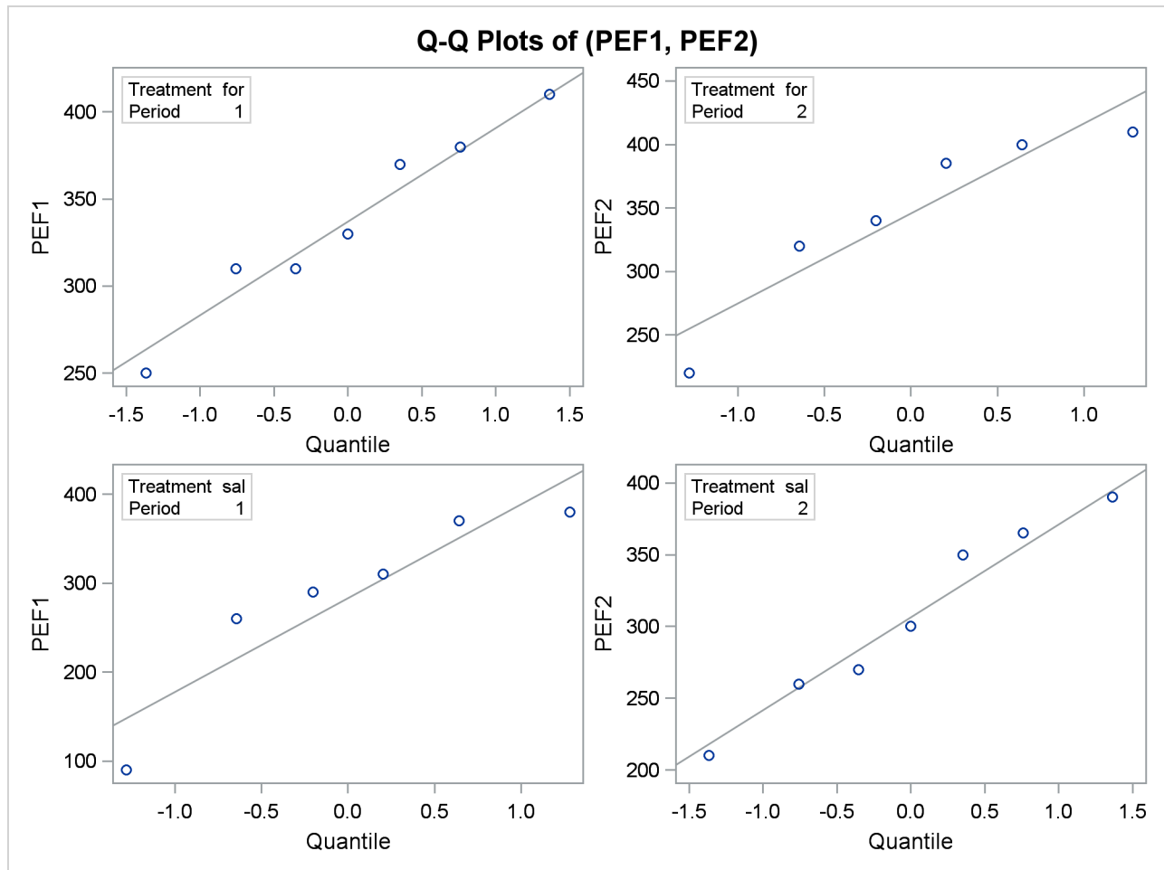
Output 119.4.11 Q-Q Plots
