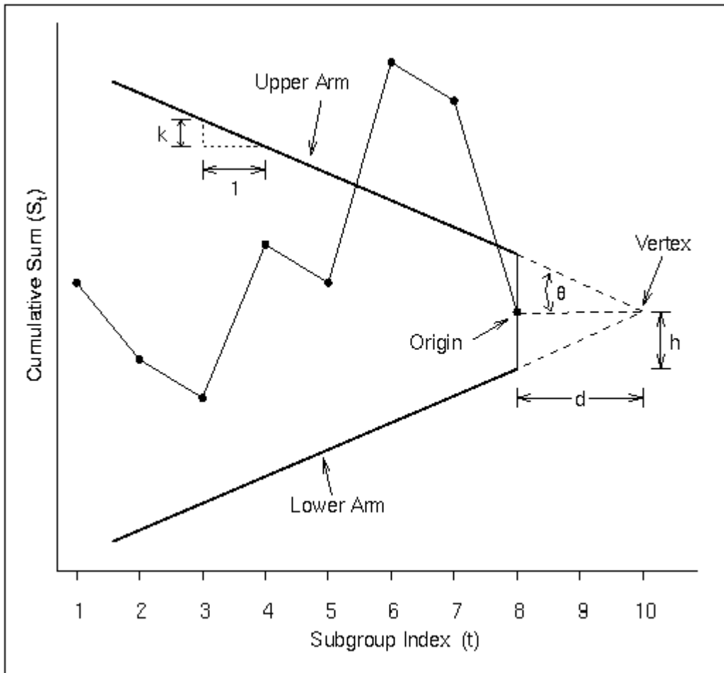
Figure 7.14 V-Mask Parameters
