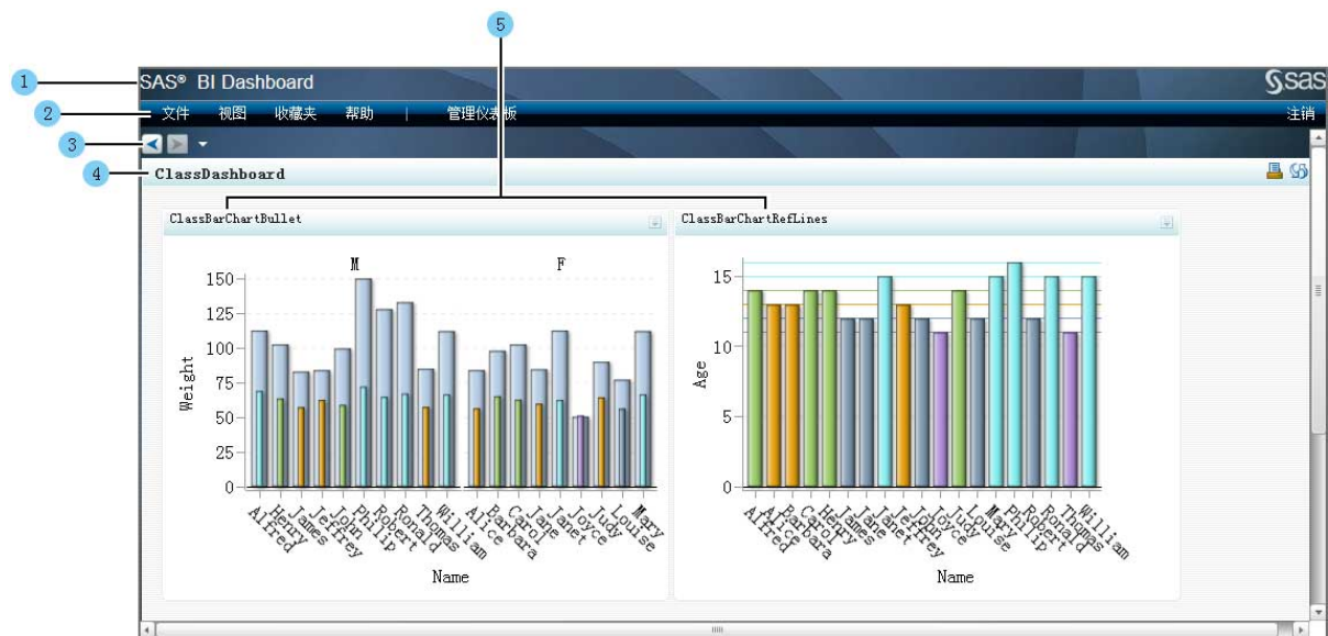
图 4.2 显示仪表板的 SAS BI Dashboard 查看器界面
