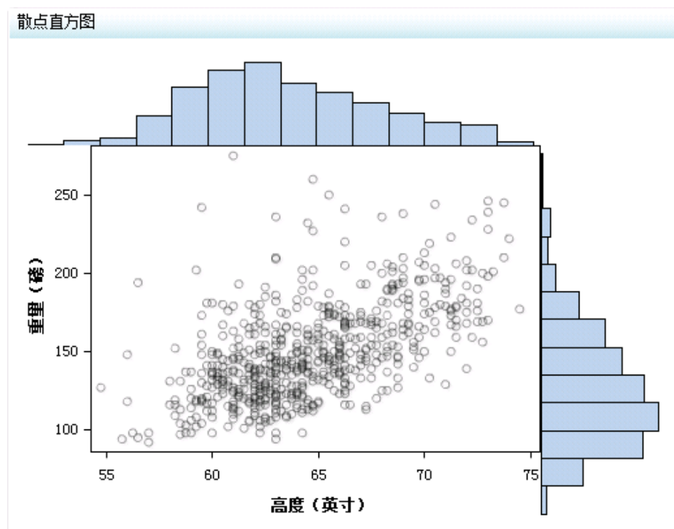
图 A1.19 散点直方图指示器示例
