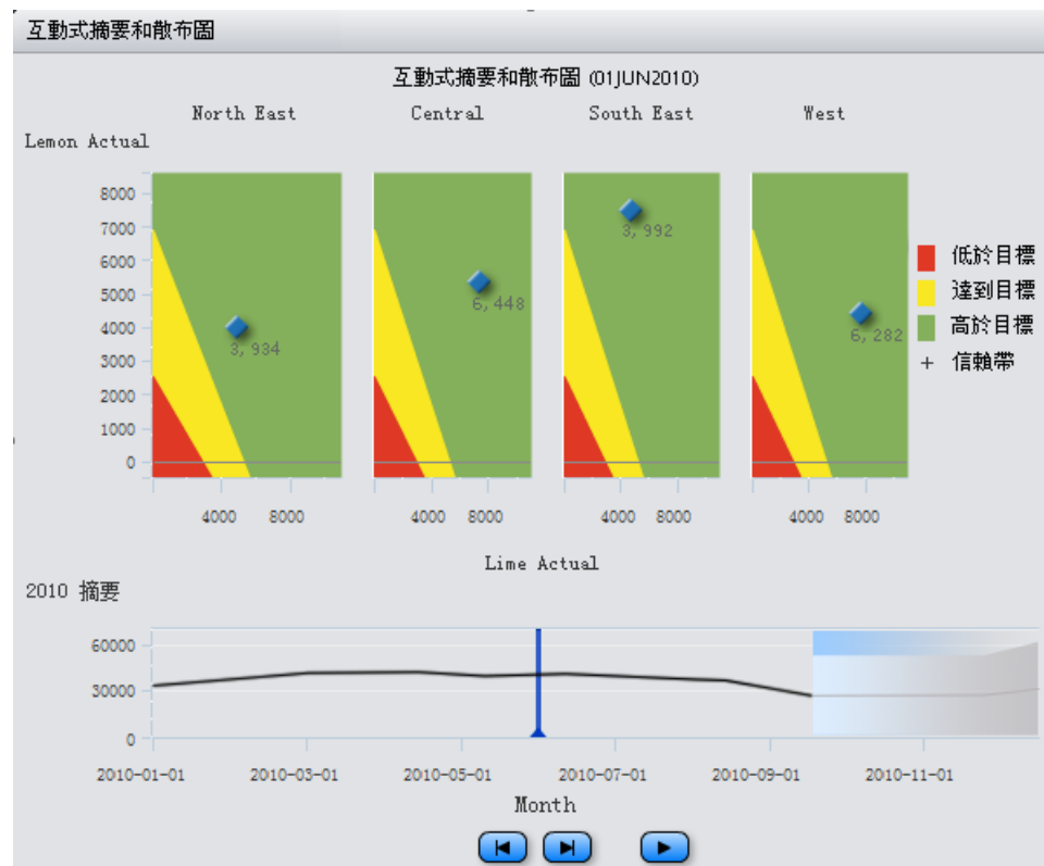
圖表 A1.12 互動式摘要和散布圖指標範例
