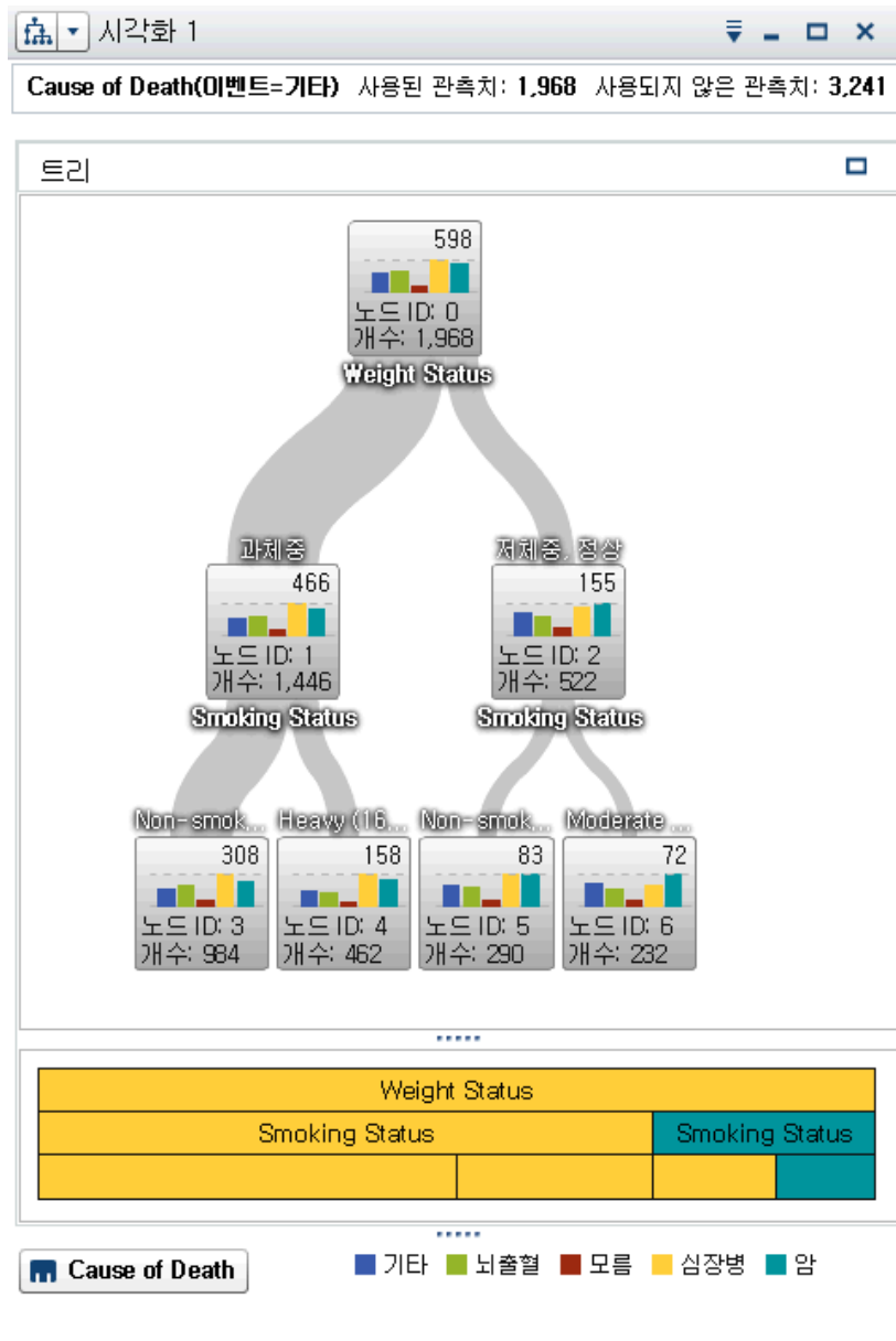
그림 25.6 의사결정트리 예
